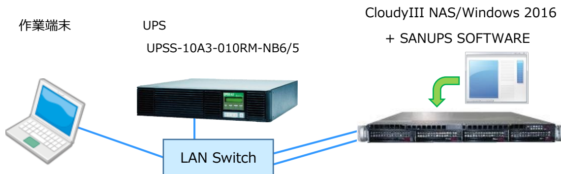
図 1. 10A3 検証構成図
