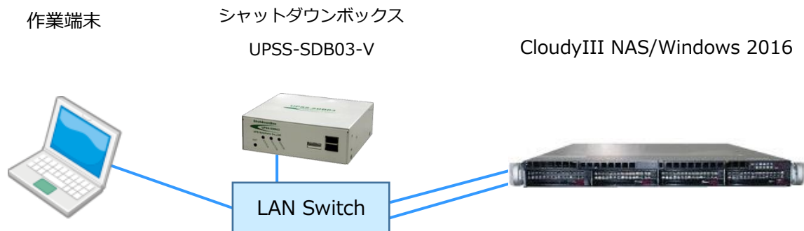
図 3. SDB03-V 検証構成図
