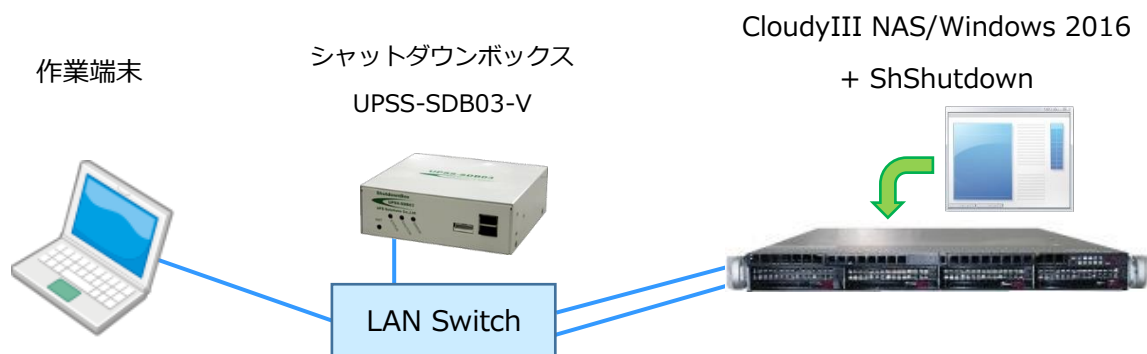
図 4. SDB03-V 検証構成図
